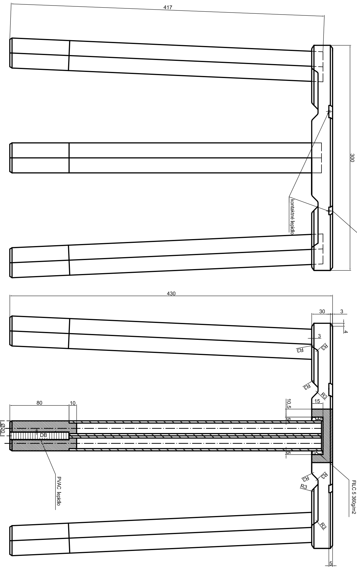
REZ A-A
